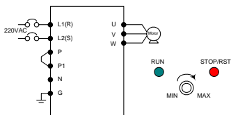
Conexión
