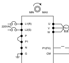
Conexionado
