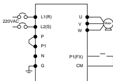
Conexión
